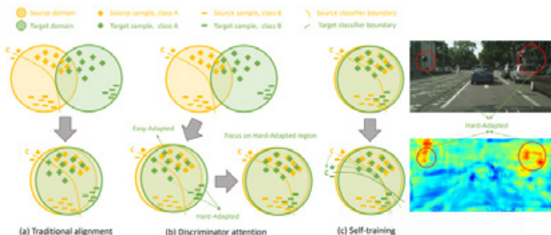
▲ 图 5 对抗学习方法
