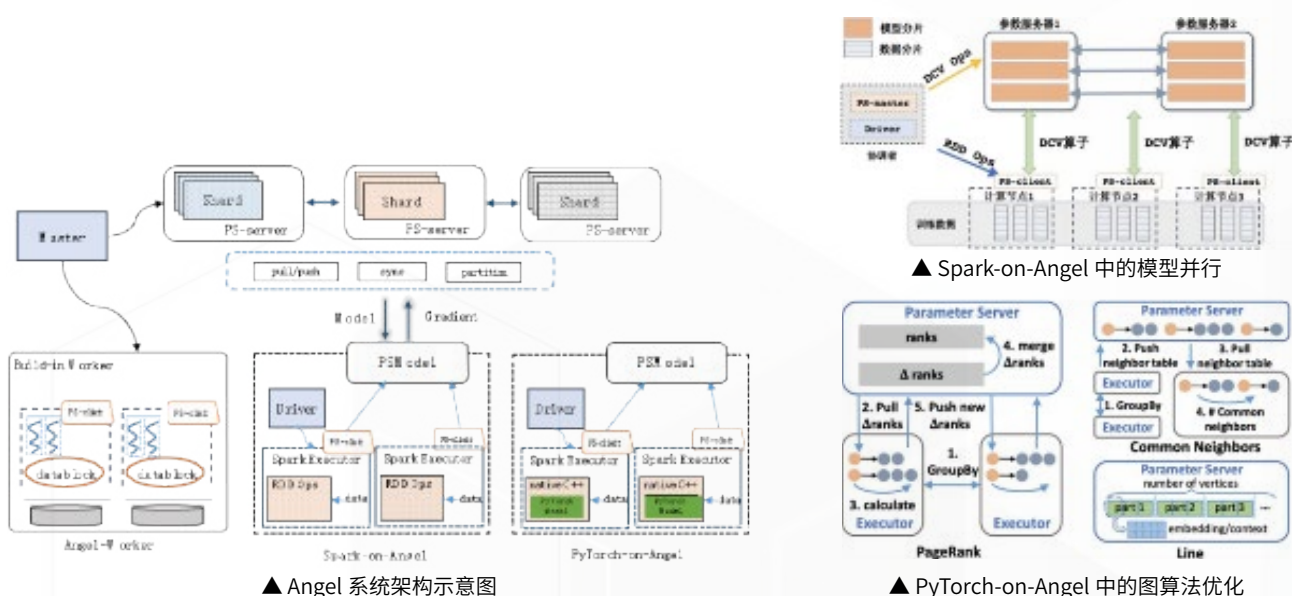
▲ Angel 系统架构示意图
