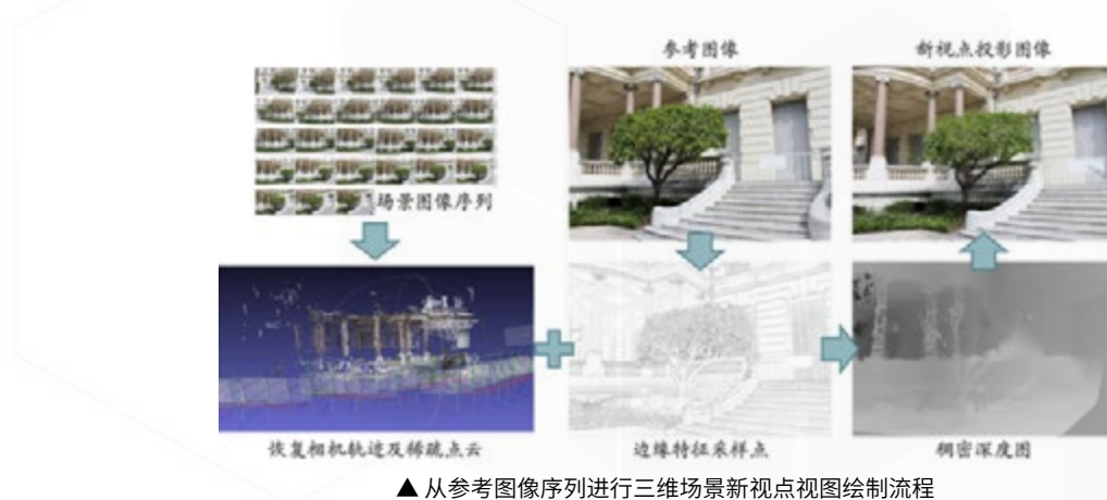
▲ 从参考图像序列进行三维场景新视点视图绘制流程
