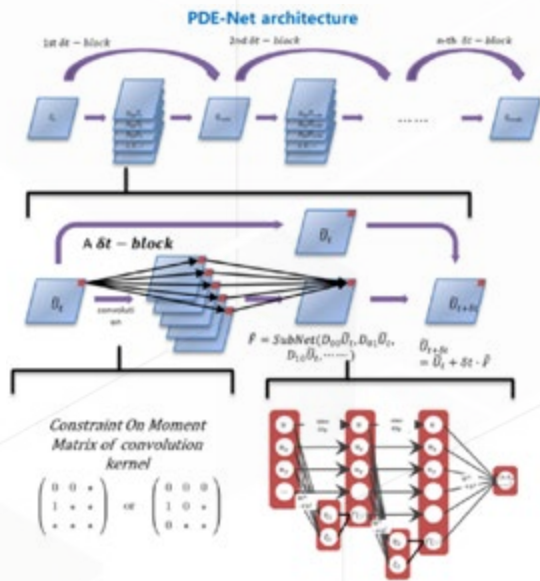
▲ 图 2 数值 PDE 算法诱导深层网络构架 Z. Long et al., ICML 2018. Z. Long, Y. Lu and B. Dong, JCP 2019.
