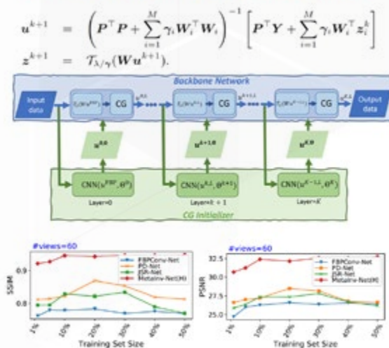
▲ 图 3 机理与数据融合的 CT 图像重建模型 H.M. Zhang et al., IEEE TMI 2021.
