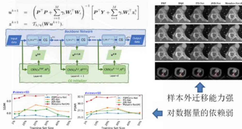
▲ 图 3 机理与数据融合的 CT 图像重建模型 H.M. Zhang et al., IEEE TMI 2021.
