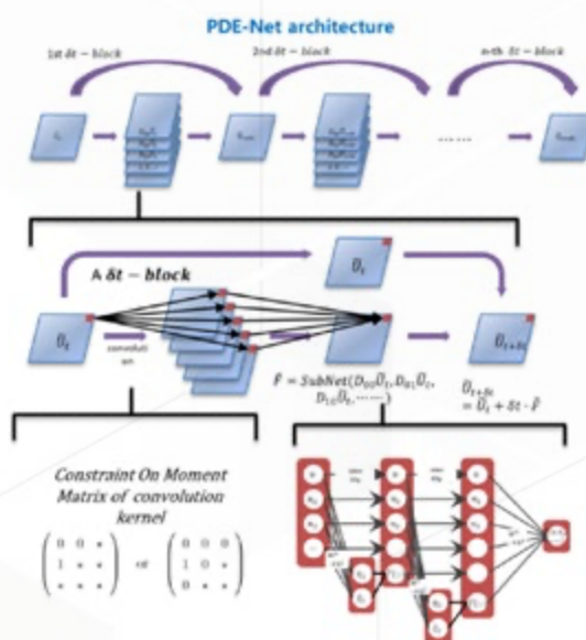
▲ 图 2 数值 PDE 算法诱导深层网络构架 Z. Long et al., ICML 2018. Z. Long, Y. Lu and B. Dong, JCP 2019.
