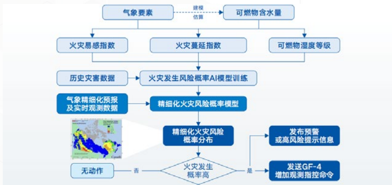
▲森林火险概率预报系统
